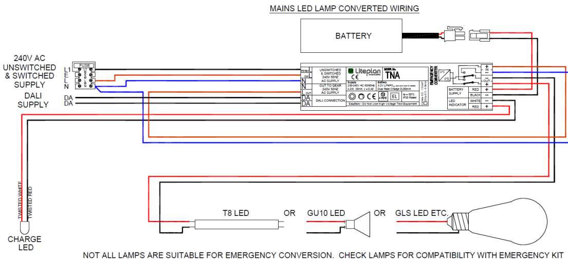
Mains Fed Lamp Wiring Diagrams
